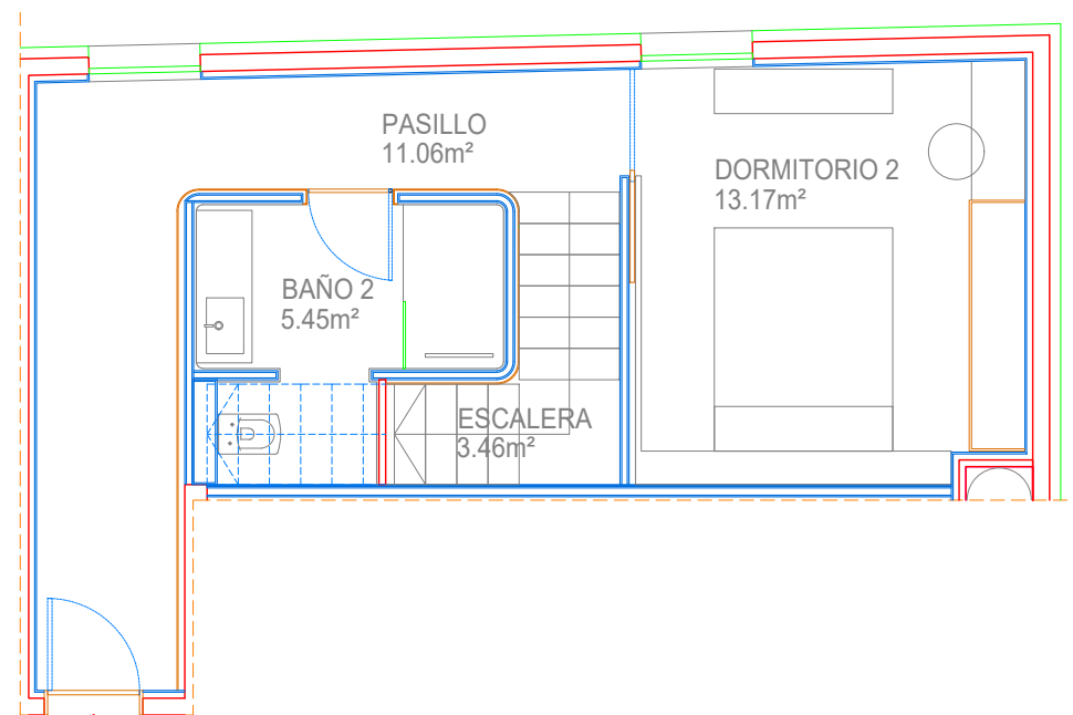
PLANTA 1ª
