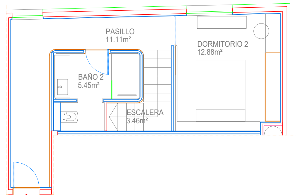
PLANTA 3ª
