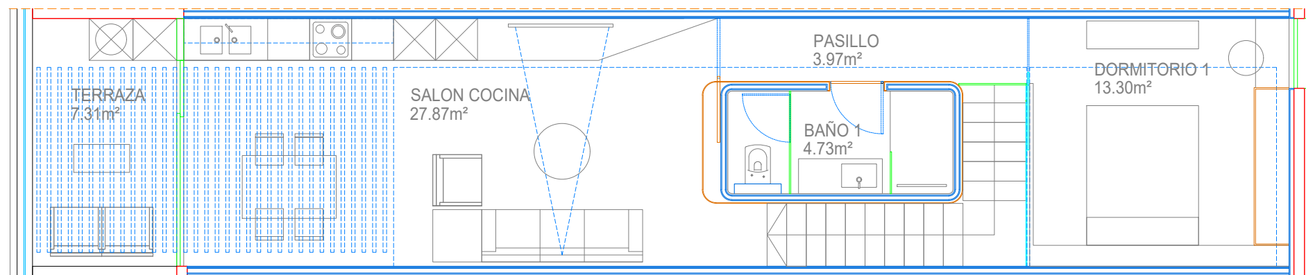
PLANTA 2ª
